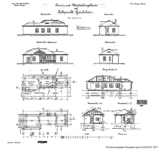
Grundrisse
