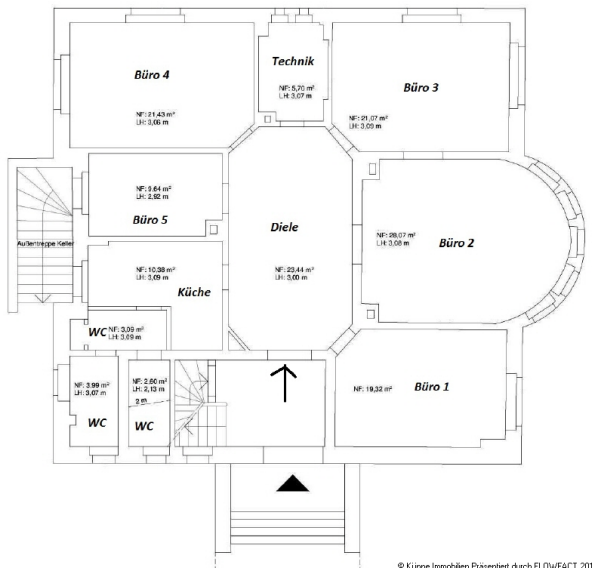
Grundriss EG
