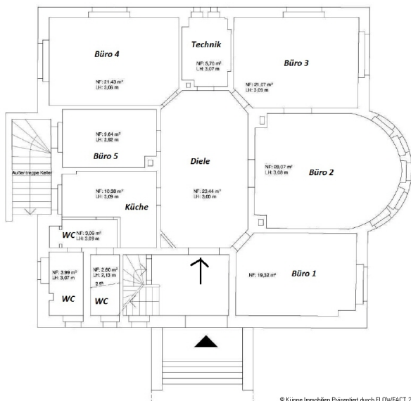
Grundriss
